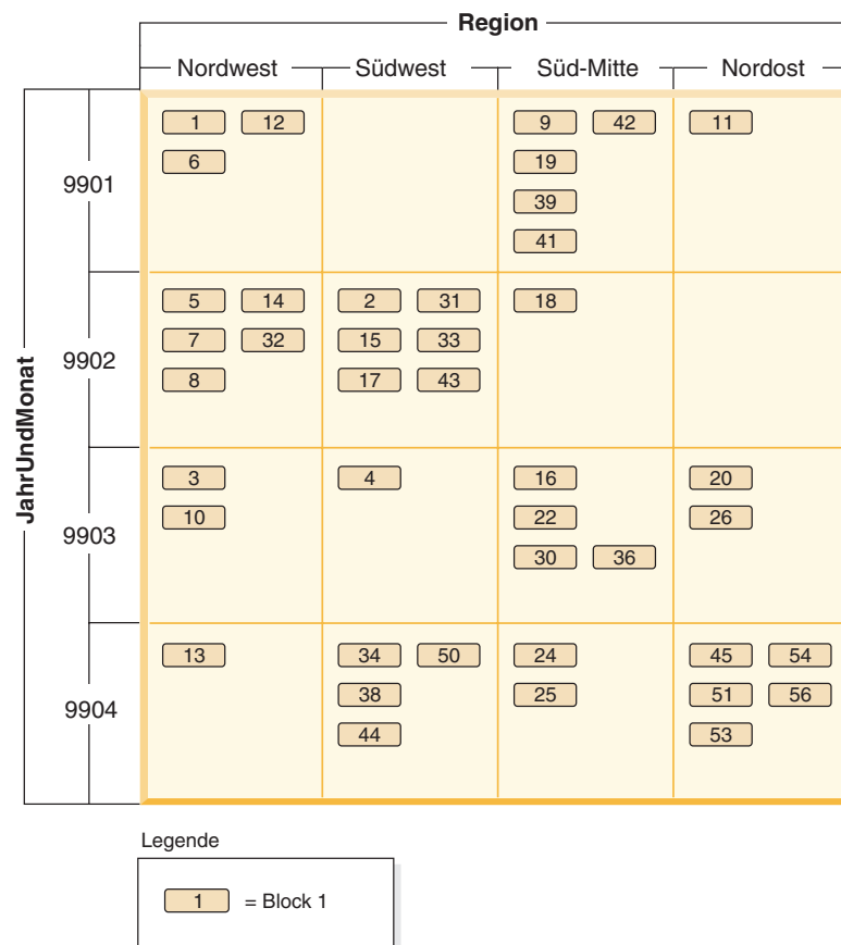
Abbildung 14. Mehrdimensionale Tabelle mit den Dimensionen 'Region' und 'JahrUndMonat' mit dem Namen 'Umsatz'
