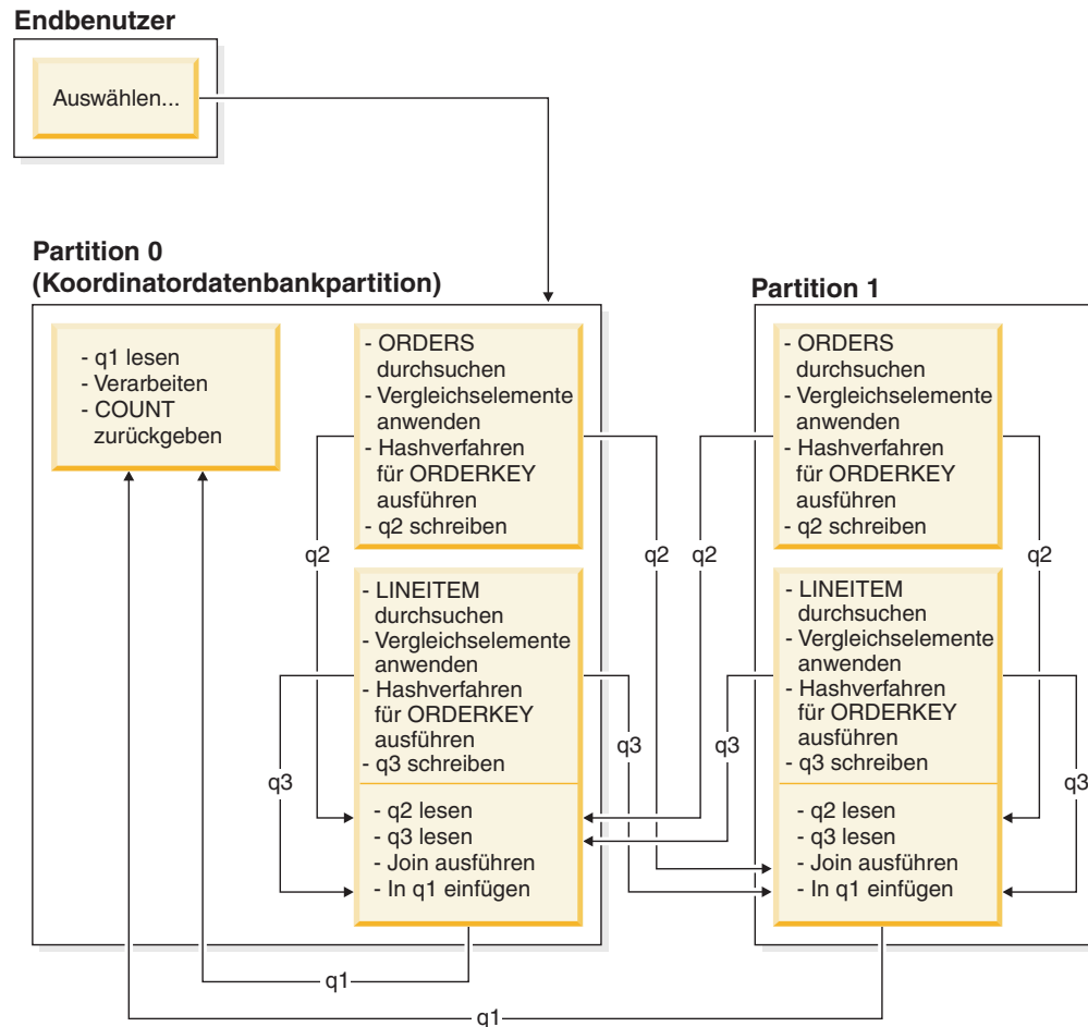
Abbildung 58. Beispiel für einen Directed-Inner-Table- und Directed-Outer-Table-Join
