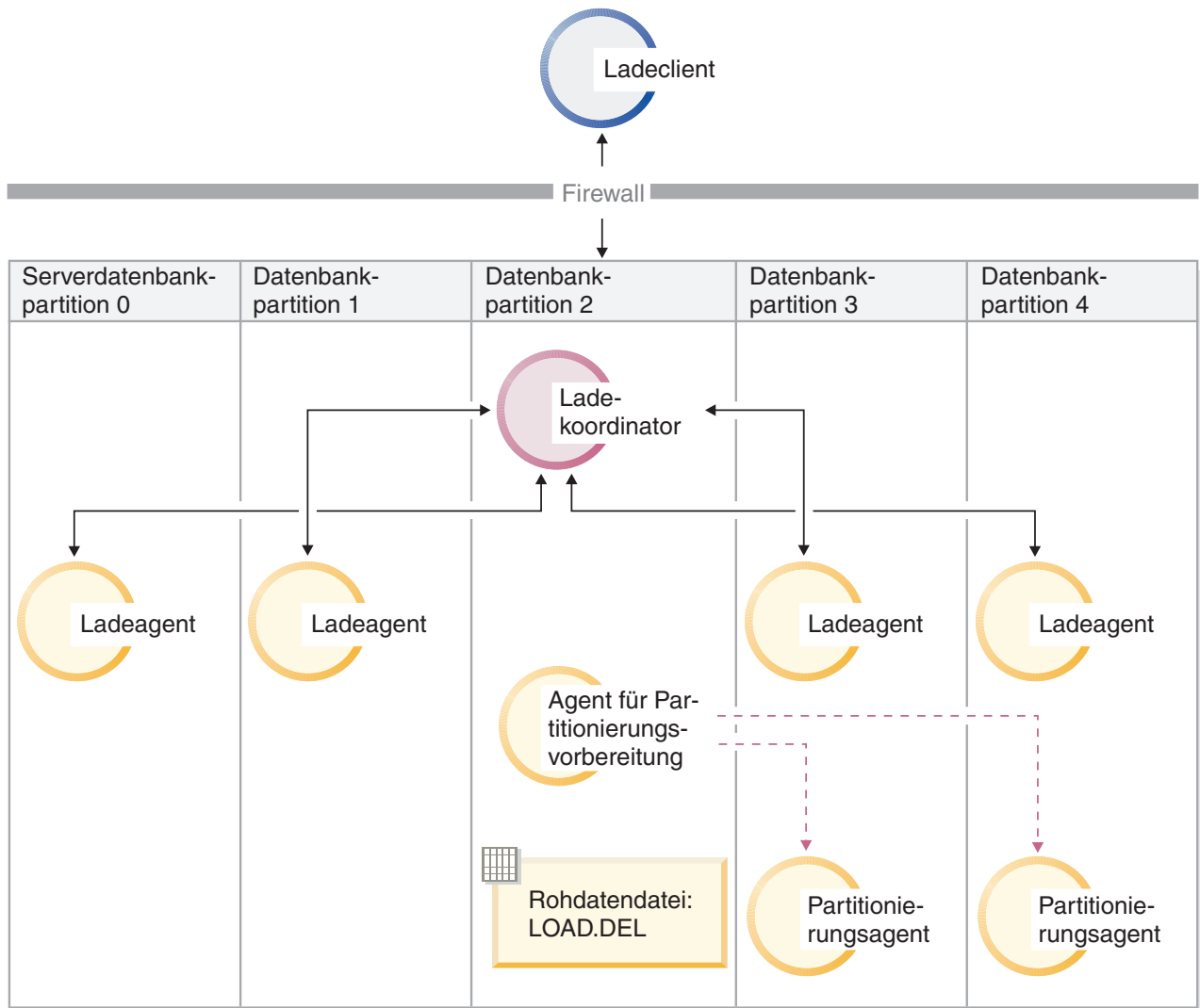
Abbildung 42. Laden von Daten in die Datenbankpartitionen 3 und 4. Diese Abbildung veranschaulicht das Verhalten, das sich bei Ausführung des vorstehenden Befehls ergibt. Die Daten werden in die Datenbankpartitionen 3 und 4 geladen.
