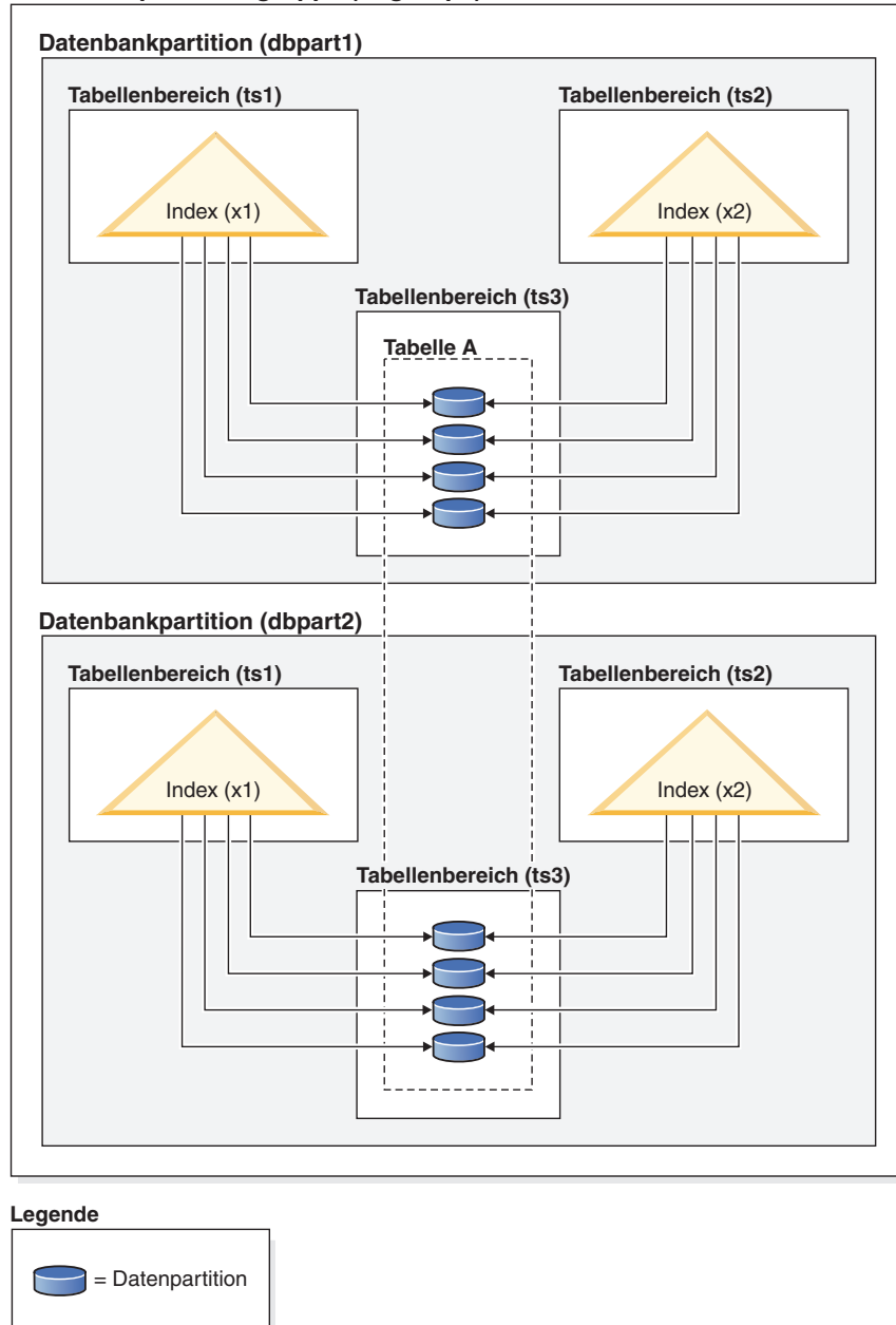
Abbildung 51. Nicht partitionierter Index für eine verteilte und partitionierte Tabelle
