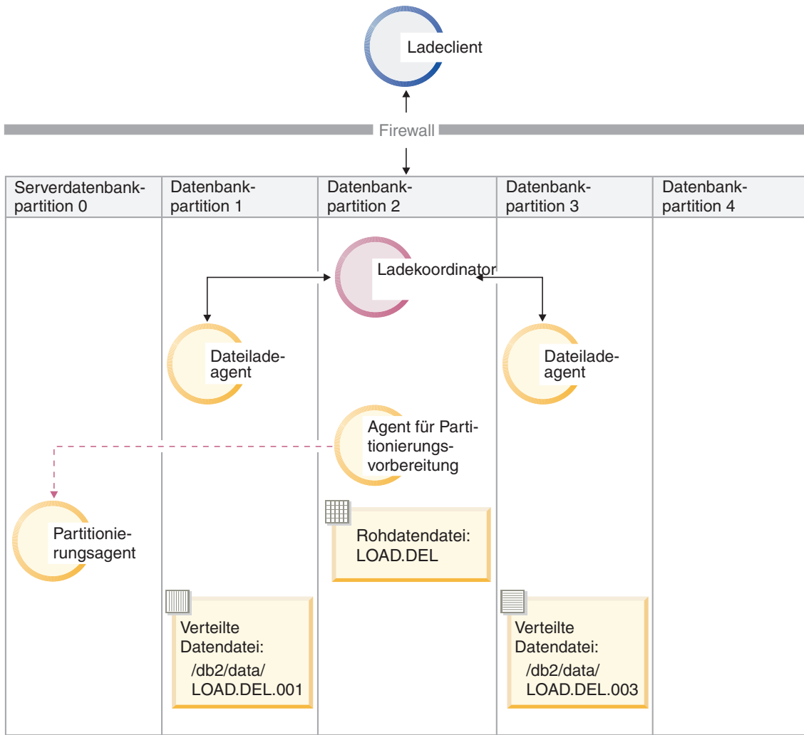
Abbildung 43. Laden von Daten in die Datenbankpartitionen 1 und 3 mithilfe eines Partitionierungsagenten. Diese Abbildung veranschaulicht das Verhalten, das sich bei Ausführung des vorstehenden Befehls ergibt. Die Daten werden auf die Datenbankpartitionen 1 und 3 geladen, wobei ein Partitionierungsagent verwendet wird, der auf Datenbankpartition 0 aktiv ist.
