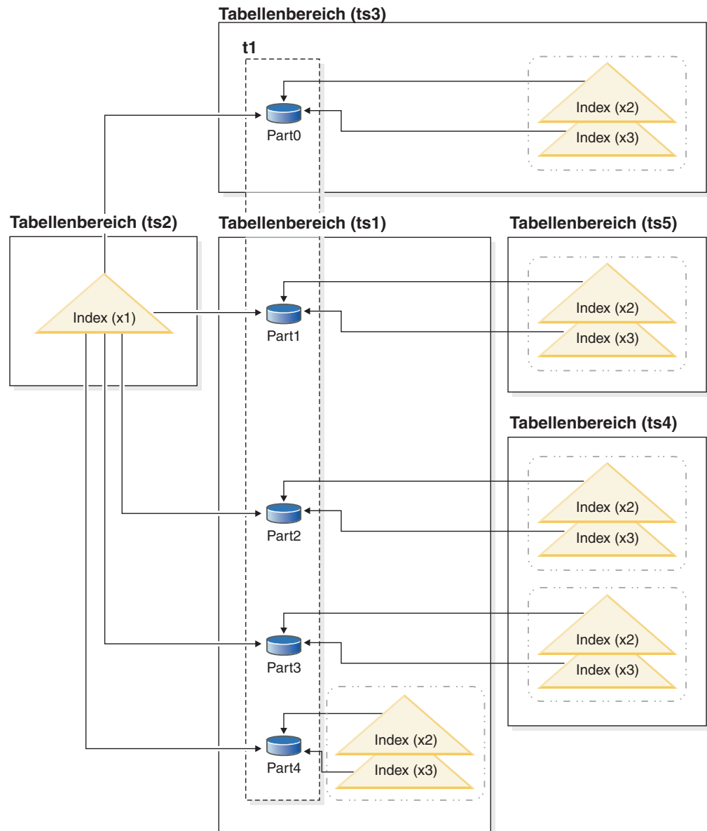
Abbildung 52. Partitionierter Index und nicht partitionierte Indizes für eine partitionierte Tabelle
