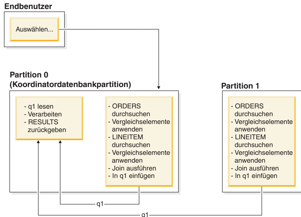
Abbildung 55. Beispiel für einen zusammengefassten Join
