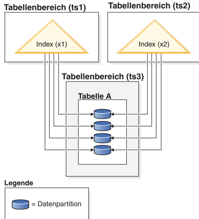
Abbildung 50. Nicht partitionierte Indizes für eine partitionierte Tabelle
