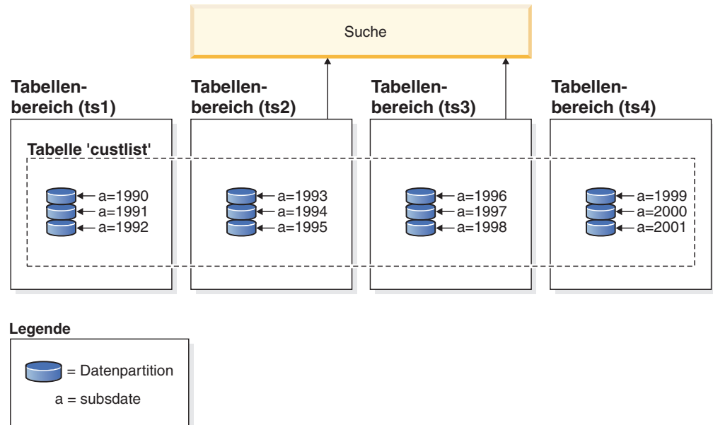
Abbildung 48. Die Leistungsvorteile des Datenpartitionsausschlusses
