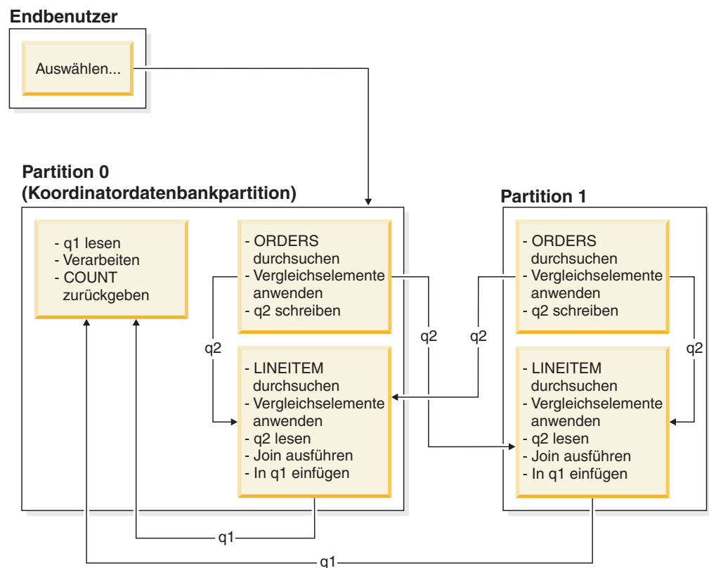
Abbildung 56. Beispiel für einen Broadcast-Outer-Table-Join
