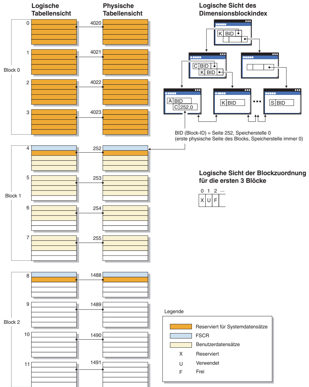
Abbildung 54. Logische Tabellen-, Datensatz- und Indexstruktur für MDC-Tabellen
