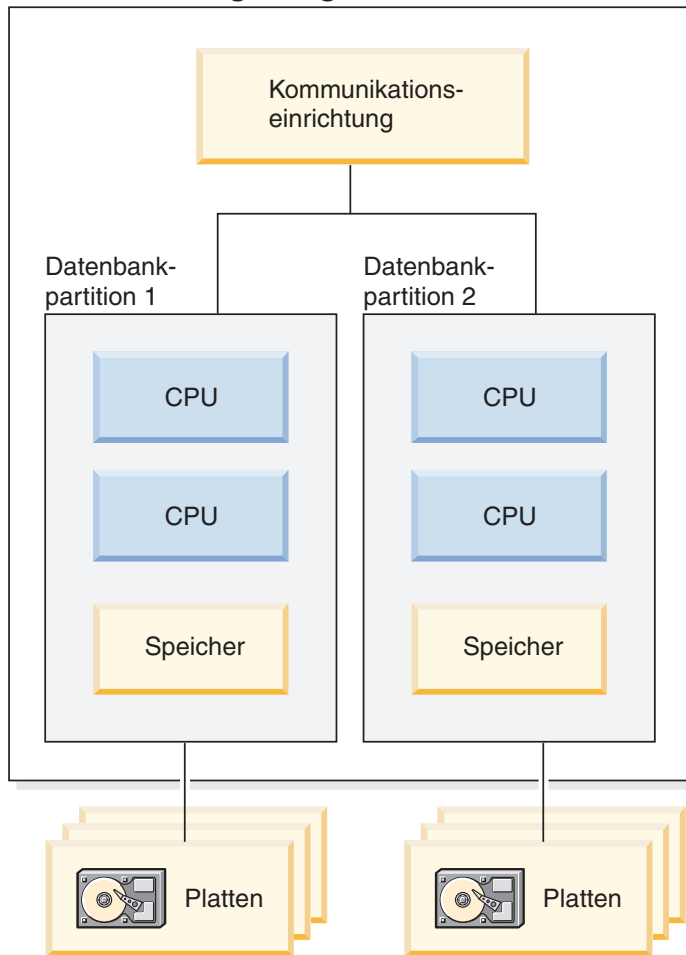
Abbildung 35. Partitionierte Datenbank mit symmetrischer Multiprozessorumgebung
